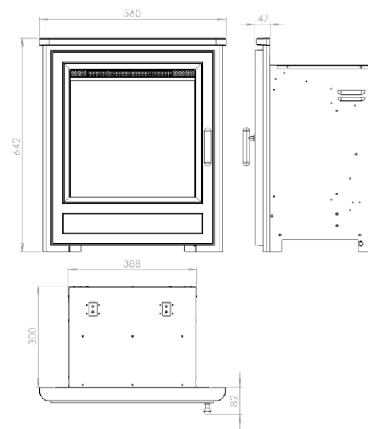
VS40 Spacer Box
