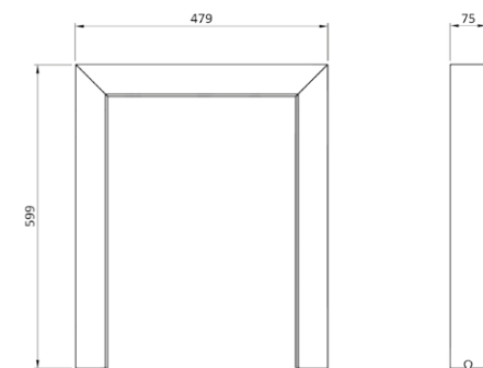
VS40 Spacer Box
